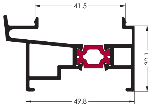
Ref. 9766 PERFIL CONDENSACION S/PT50
