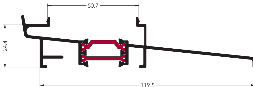
Ref. 9729 PERFIL CONDENSACION S/PT60
