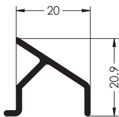
Ref. 1607 VIERTEAGUAS
