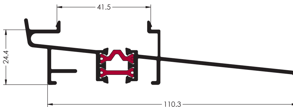
Ref. 9727 PERFIL CONDENSACION S/PT50
