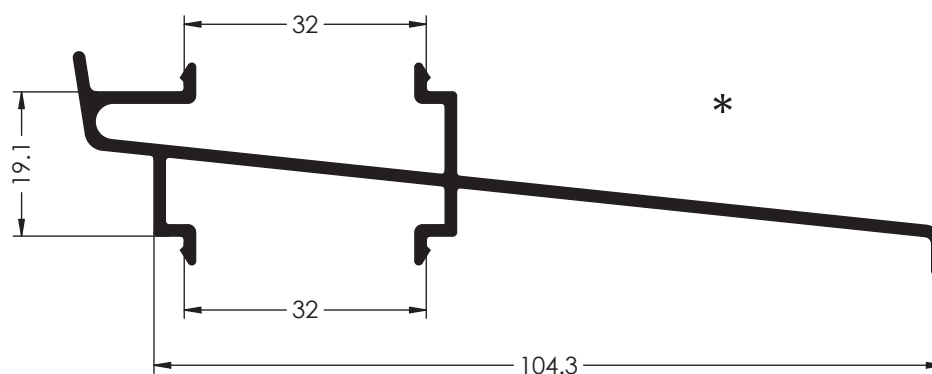
Ref. 1658 PERFIL CONDENSACION S/PRACTIC
