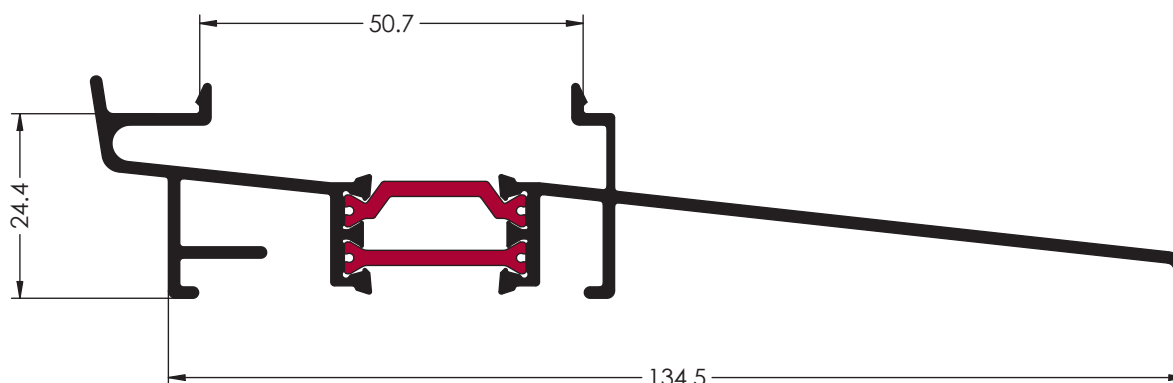
Ref. 9747 PERFIL CONDENSACION S/PT60
