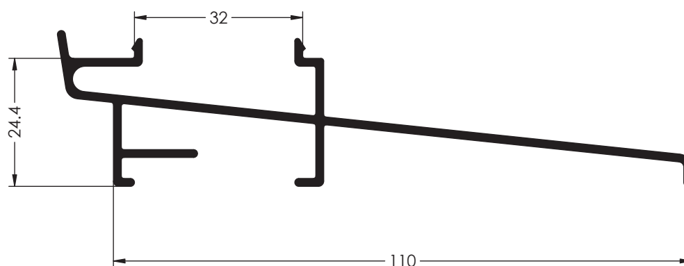
Ref. 1713 PERFIL CONDENSACION S/PRACTIC
