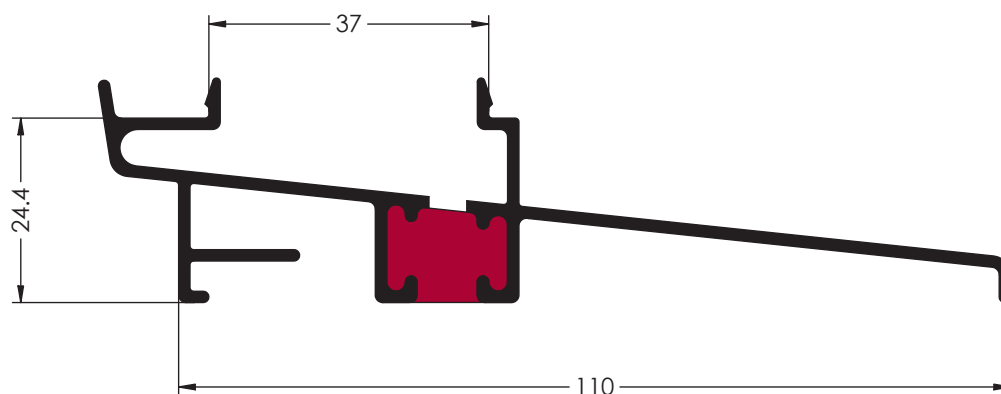
Ref. 9650 PERFIL CONDENSACION S/TERMIC
