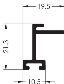
Ref. 1716 CORTAVIENTOS PUERTAS
