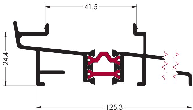
Ref. 9746 PERFIL CONDENSACION S/PT50
