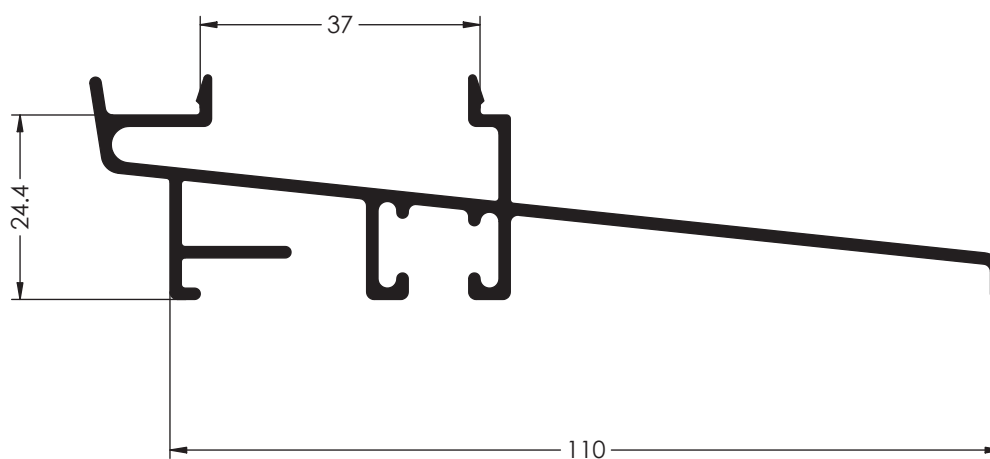
Ref. 1714 PERFIL CONDENSACION S/CLASIC Y S/PRACTIC45
